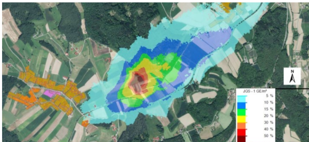
Beispiel für ein Geruchsfahnenberechnung nach GRAL (Grundlagen für die Modellierung der Geruchsausbreitung aus der Tierhaltung mit dem Lagrange'schen Partikelmodell GRAL)
